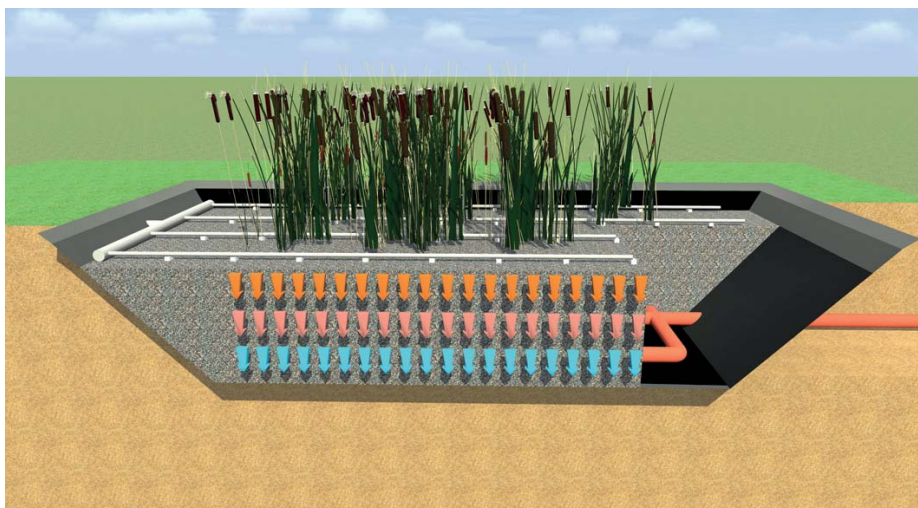
Schéma vertikálního kořenového filtru – přítokové potrubí rozložené na povrchu (šedá barva), sítěná drenáž ve spodní části (oranžová), voda protéká převážně ve vertikálním směru
